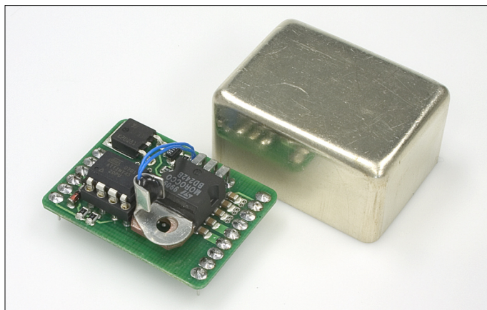
Bild 1: Die mit allen SMD-Bauteilen fertig bestückte Platine
