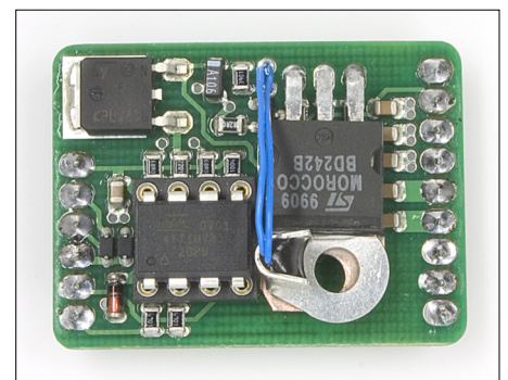
Bild 5: vollständig bestückte Platine; der Si570 ist vor dem Aufkleben des Heiztransistors anzuschleifen. Die Stiftleisten werden von unten bestückt.
