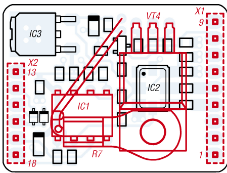
Bild 3: Bestückungsplan der Synthesizer-Platine; nur die rot markierten Bauteile sind noch einzulöten, die schwarz dargestellten SMD-Bauteile sind im Bausatz schon aufgelötet. Abmessung 34,5 mm x 25,7 mm, nicht maßstäblich. Die beiden Stiftleisten haben das Rastermaß 2,54 mm, ihr Abstand beträgt 30,48 mm. (siehe auch Abschnitt 7)
